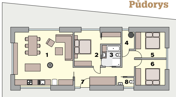
1 obytný prostor s kuchyní, 2 ložnice se šatnou, 3 koupelna, 4 technická místnost, 5 + 6 ložnice, 7 předsíň, 8 WC
